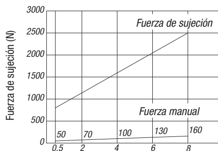
Sujeción por tracción 04400-4050...
