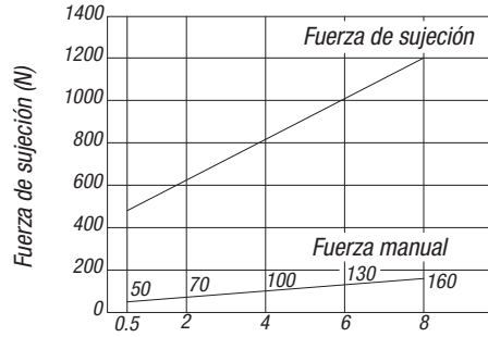
Dispositivo de sujeción pivotante 04366-...4540
