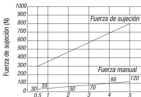
Dispositivo de sujeción pivotante 04366-...3232
