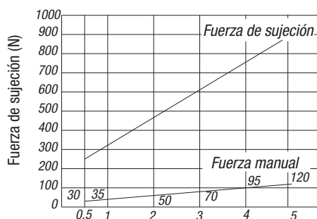
Sujeción por tracción 04400-3240...
